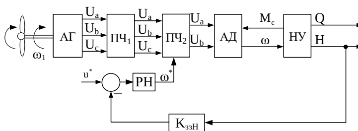
Рис. 1. Функціональна схема досліджуваної системи
