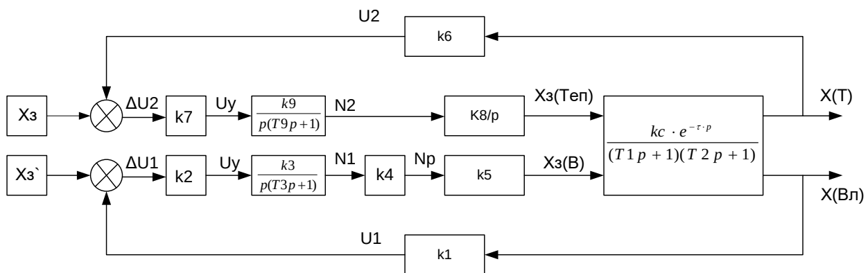
Рис. 1. Структурна схема САК камери копчення
