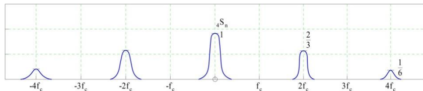
Рис. 3 Спектральна щільність відносних величин різних смуг спектра
