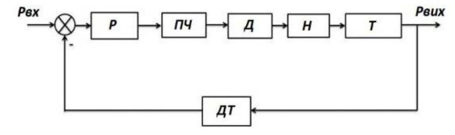
Рис. 1. Структурна схема САК тиском в подаючому трубопроводі: Р – регулятор, ПЧ – перетворювач частоти, Д – електродвигун, Н – насос, Т – трубопровід, ДТ – датчик тиску
